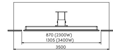
MINIMALE UITSPARING OPTIE 2 2300/3400W
