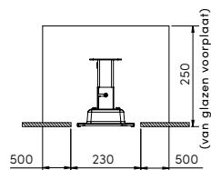
UITSPARINGSKIT VOOR MINDER VRIJE RUIMTE 2300/3400W
