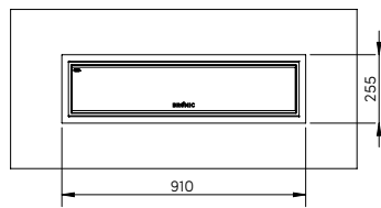
MINIMALE UITSPARING OPTIE 1 2300/3400W
