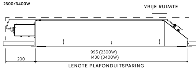
UITSPARINGSKIT VOOR MINDER VRIJE RUIMTE 2300/3400W
