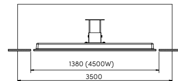
MINIMALE UITSPARING VOOR 4500W
