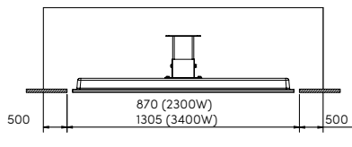
MINIMALE UITSPARING OPTIE 1 2300/3400W
