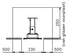
UITSPARINGSKIT VOOR MINDER VRIJE RUIMTE 2300/3400W
