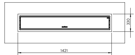
MINIMALE UITSPARING VOOR 4500W
