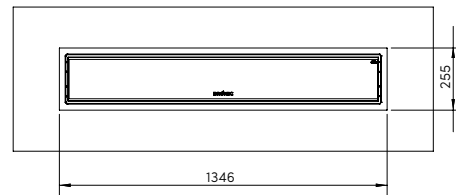
MINIMALE UITSPARING OPTIE 2 2300/3400W
